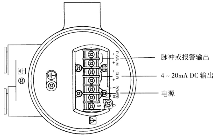
一体型接线端子位置
