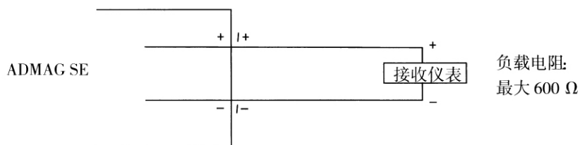
模拟信号输出连接
