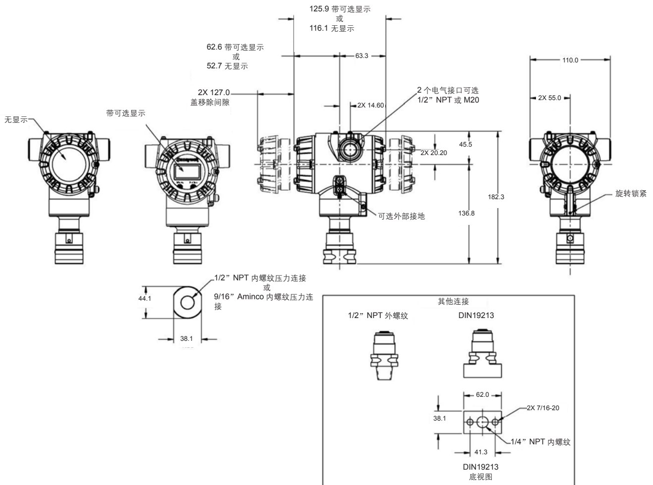
图 4 STG73L / STG73S / STG74L / STG74S / STG77L / STG77S / STG78L / STG78S / STG79L / STG79S 典型安装尺寸图
