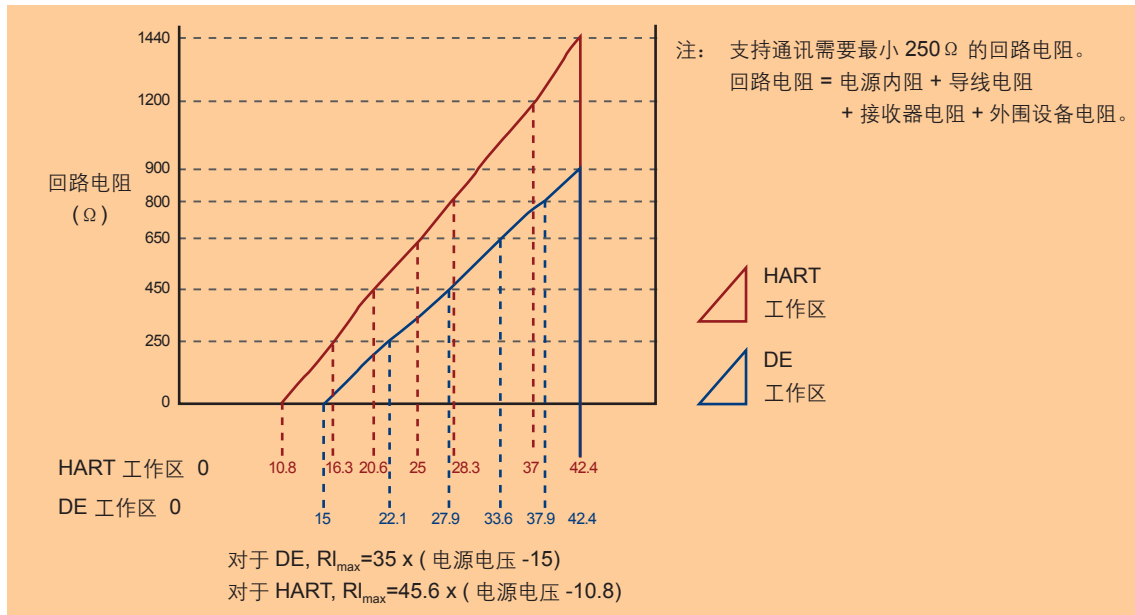
图 2 电源电压和回路电阻图以及计算
