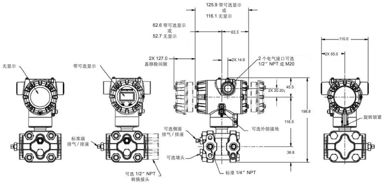
图 3 STG730 / STG735 / STG740 / STG745 / STG770 / STG775 典型安装尺寸图
